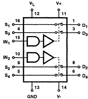
DIP (JE, PE) DUAL DPST IH5145
