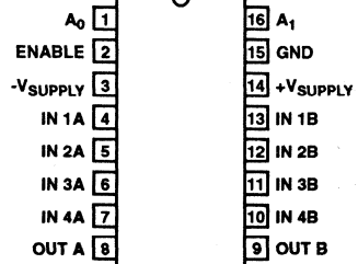
HI1-509A (CDIP) HI3-509A (PDIP) TOP VIEW
